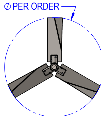
SECTION A-A: IMPELLER DETAIL
